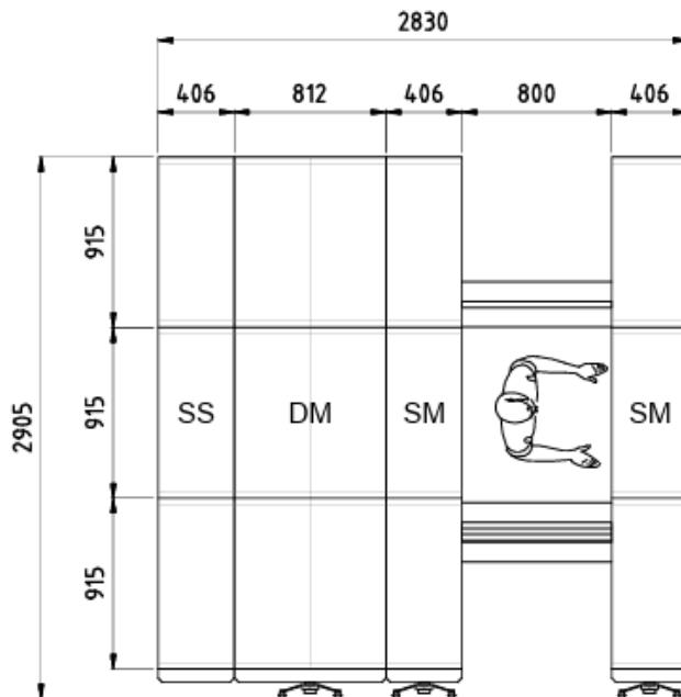
TOP ELEVATION
