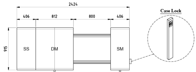
TOP ELEVATION
