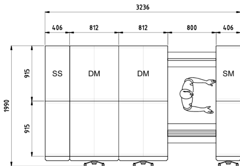
TOP ELEVATION
