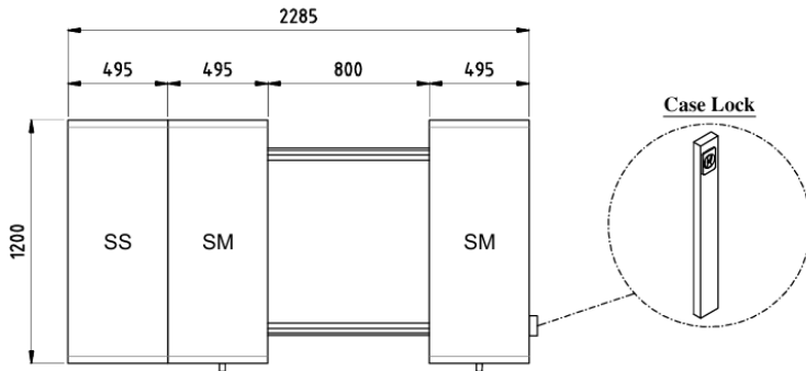
TOP ELEVATION
