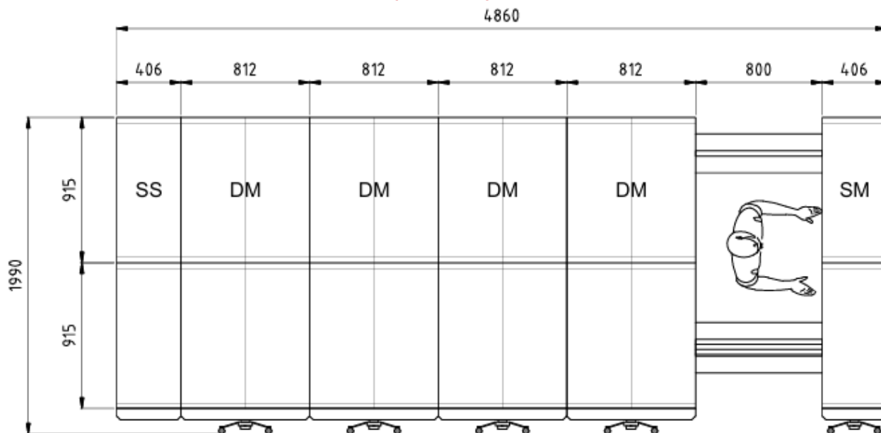
TOP ELEVATION
