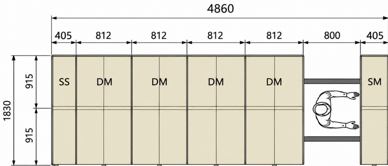
TOP ELEVATION
